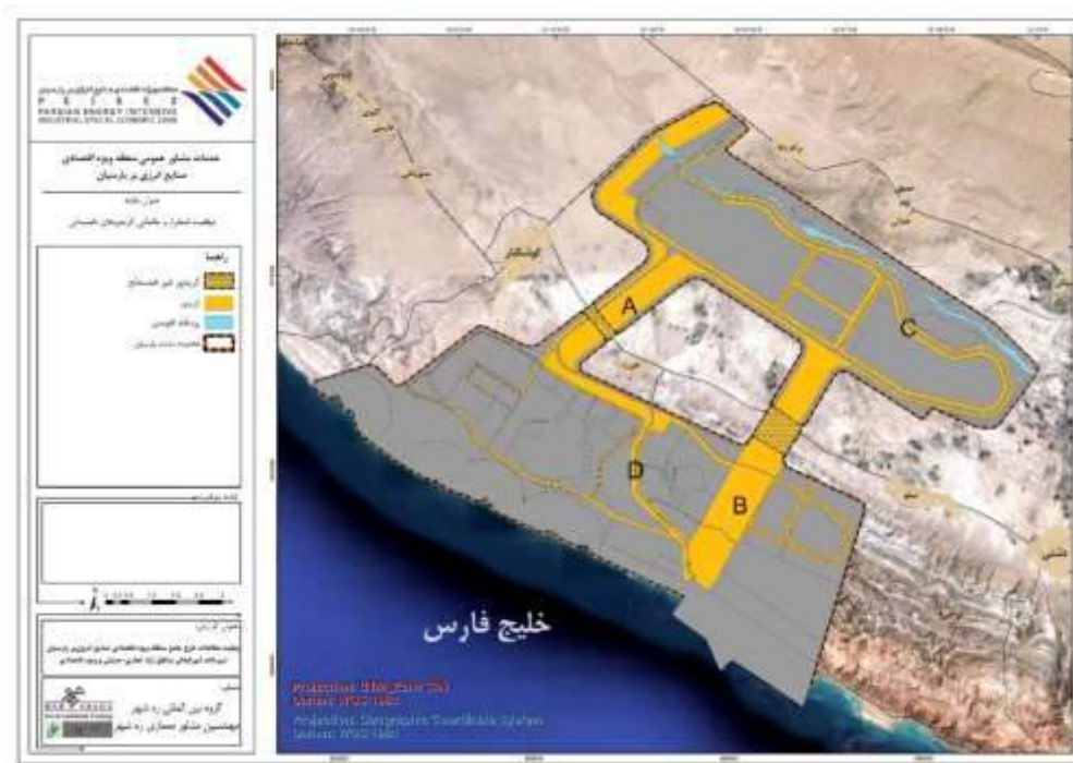
نقشه ۴- شبکه کریدورهای تأسیساتی پیشنهادی در طرح جامع منطقه ویژه اقتصادی صنایع انرژی‌بر پارسیان برگرفته از: گزارش «جمع‌بندی و تلفیق مطالعات پایه» به شماره سند ۰۰۳۲۰۰ RP O ۰۲۷۴۱، گروه بین‌المللی ره‌شهر-۱۳۹۵
