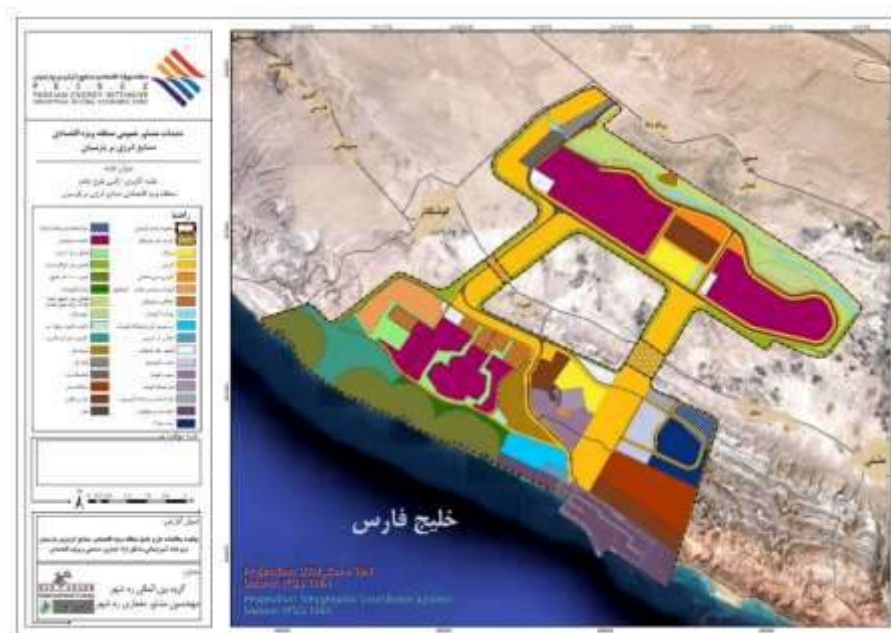
نقشه ۷- کاربری اراضی طرح جامع منطقه ویژه اقتصادی صنایع انرژی بر پارسیان برگرفته از: گزارش «جمع بندی و تلفیق مطالعات پایه» به شماره سند ۰۰۳۲۰۰ RP ۰۴۰۲۷۴۱، گروه بین المللی رهشهر-۱۳۹۵. جدول ۱۰- مساحت کاربری اراضی در طرح جامع منطقه ویژه اقتصادی صنایع انرژی بر پارسیان
